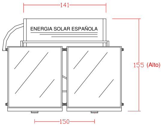
ALZADO
